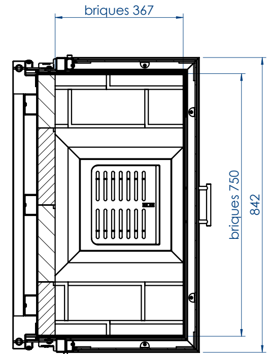
COUPE D-D
