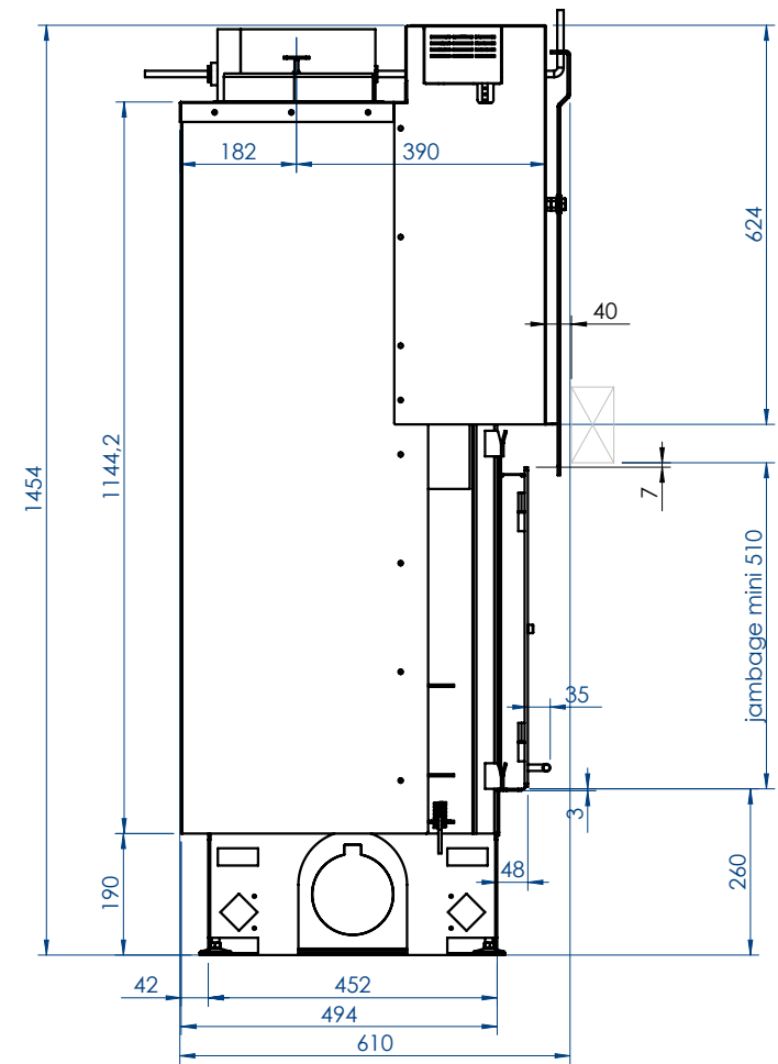
COUPE A-A
