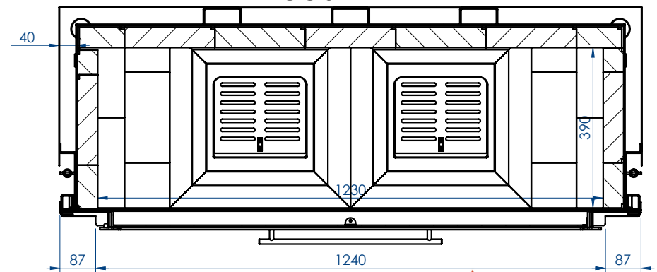
COUPE A-A
